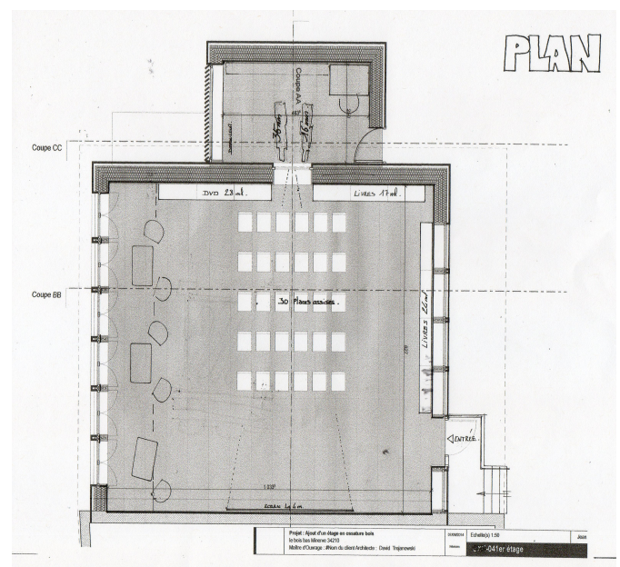
Projet de création d'un étage, à ossature bois, pour une bibliothèque, salle de lecture et cinéma avec cabine de projection.
